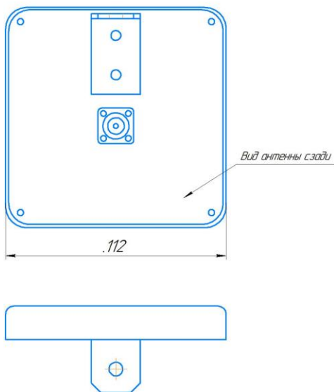
Антенна DS2400-11 (стандартная модификация)
